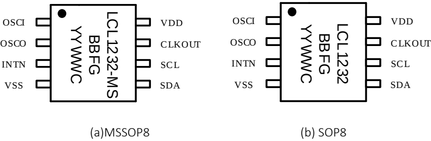
图 5-1 LCL1232 封装形式
