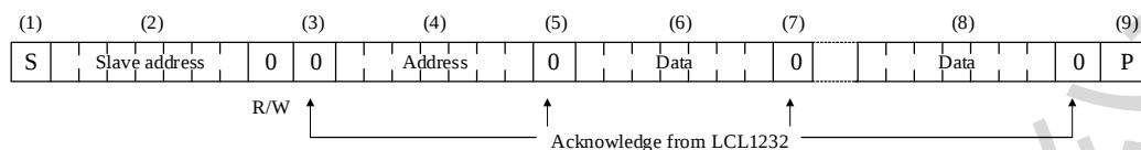
图 12-4 指定地址写操作
