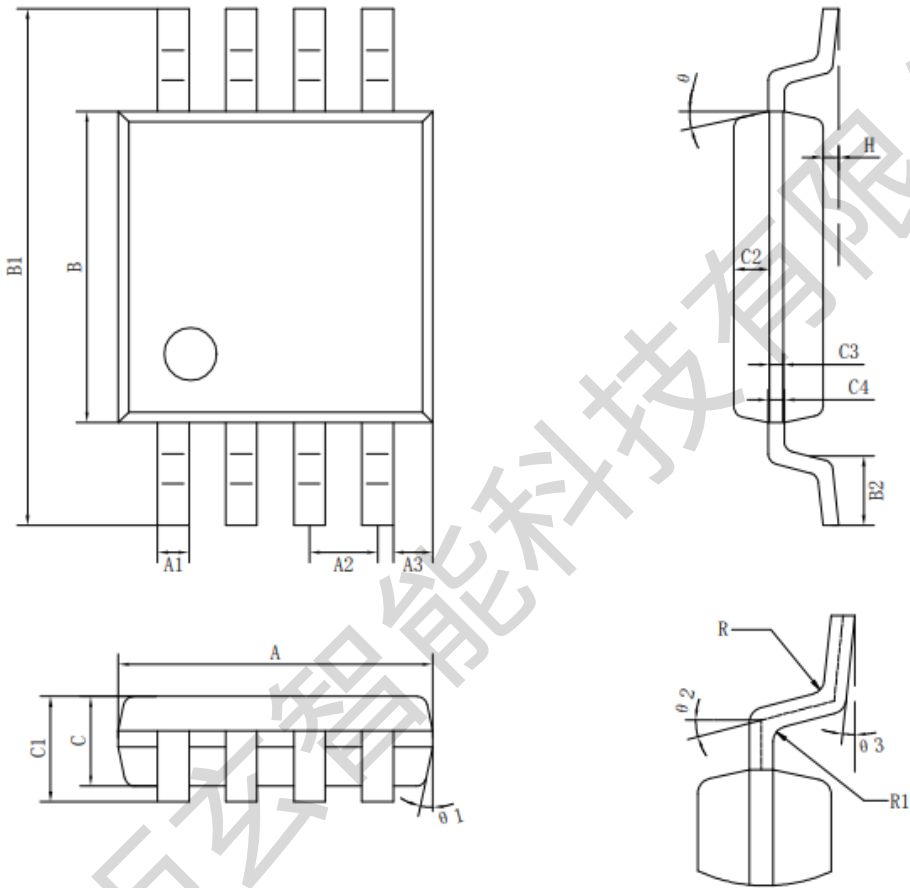
MSSOP 封装尺寸
