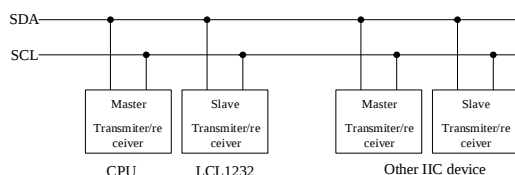
图 12-3 IIC 系统配置
