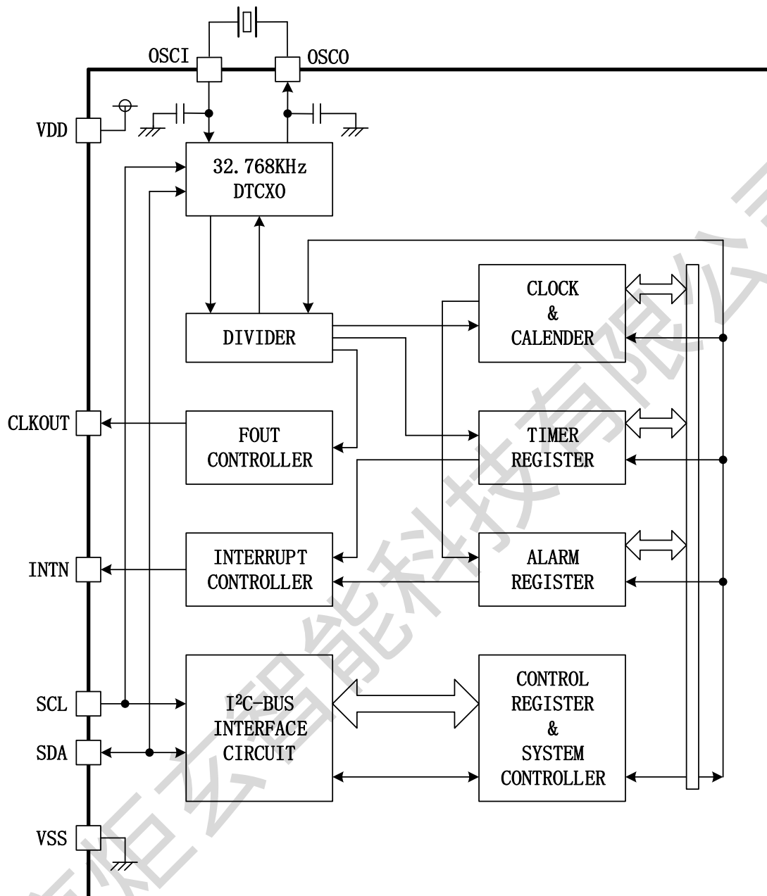
图 4-1 LCL1232 系统框图
