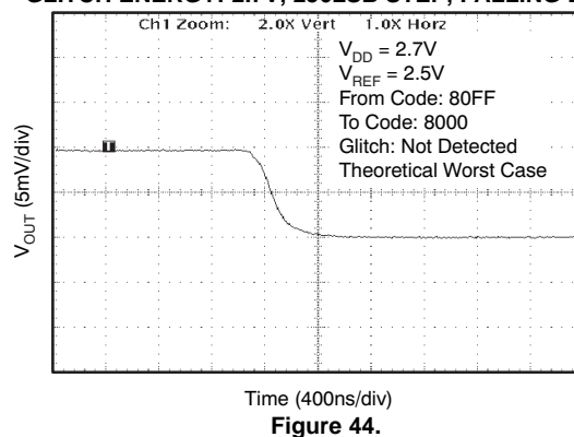
GLITCH ENERGY: 2.7V, 256LSB STEP, FALLING EDGE
