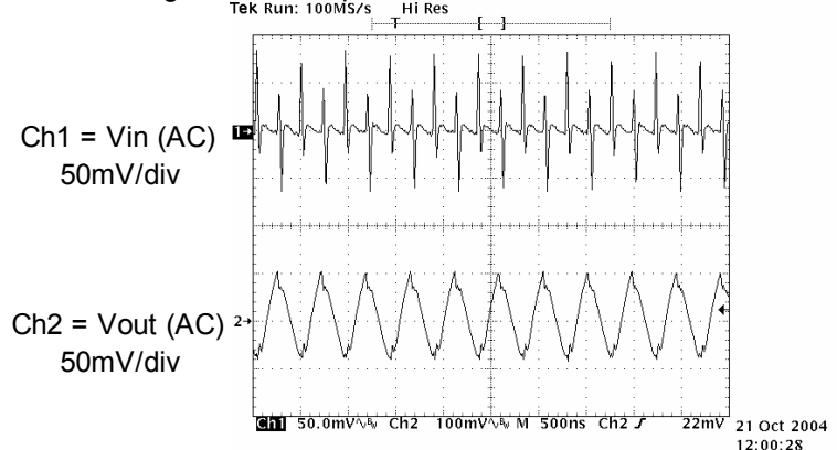
Figure 8. Ripple 700mA Flash, Vin=3.6V, Vout=3.35V.
