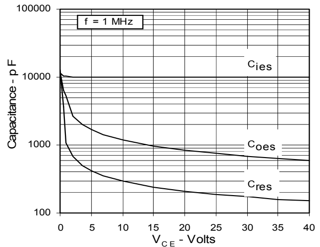
Fig. 12. Capacitance
