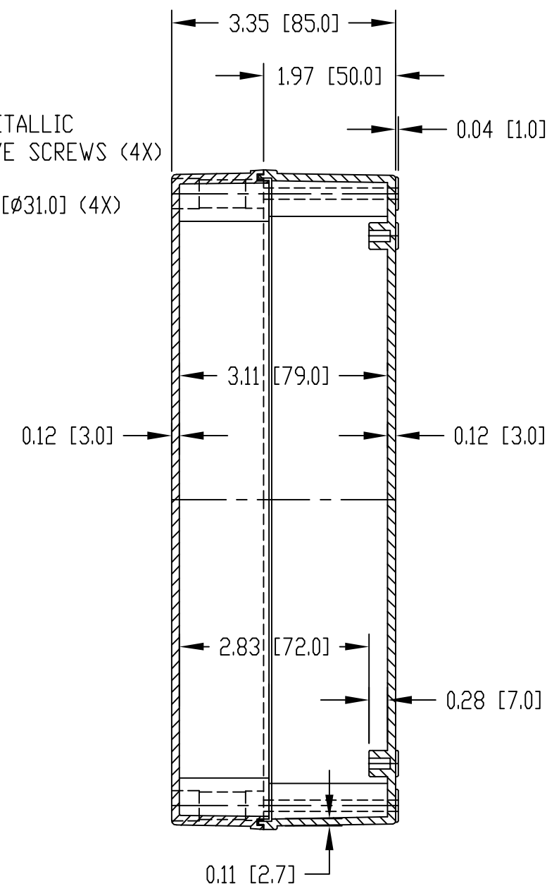
SECTION A-A
