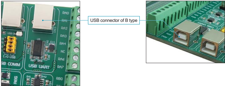
Figure 14-1: USB UART module
