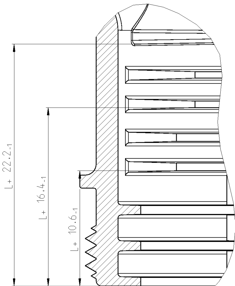
SECTION A-A Schnitt SCALE 5:1 Maßstab
