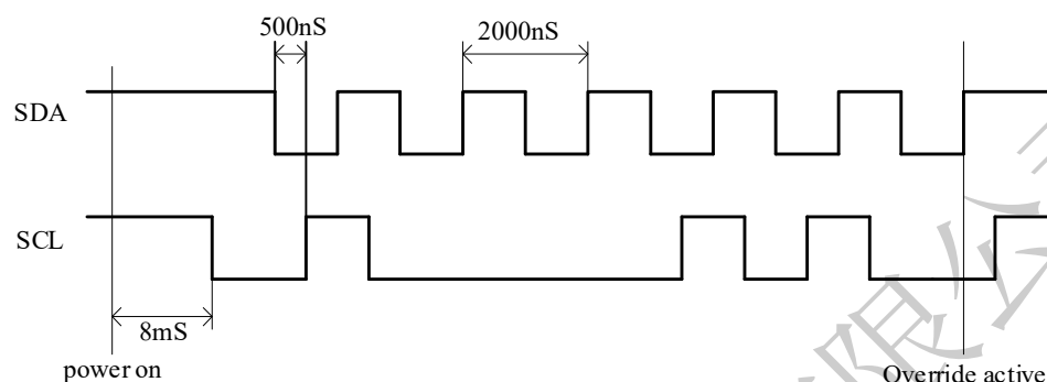
图 10-2 POR 屏蔽功能启动时序
