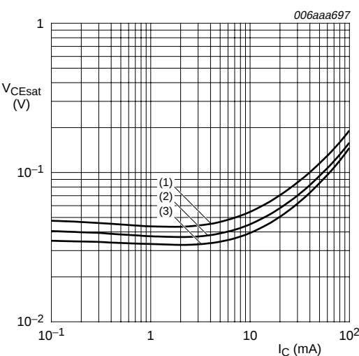
I C /I B = 20 (1) T amb = 100 °C (2) T amb = 25 °C (3) T amb = -40 °C
