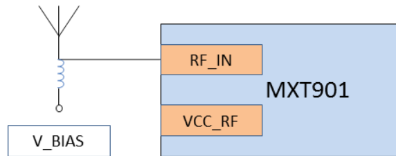
图 9-2 MXT901 其他电压范围的有源天线方案
