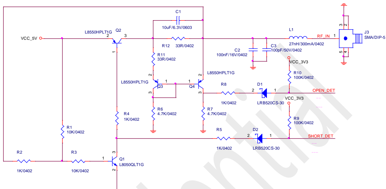
图 9-6 MXT901 天线检测参考电路
