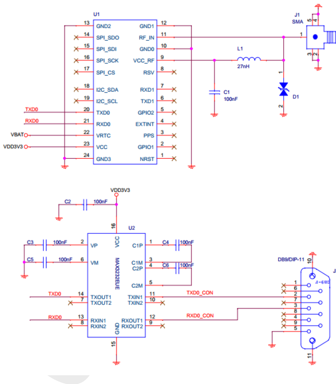
图 9-5 MXT901 最小参考设计原理图
