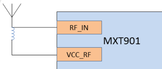
图 9-1 MXT901 3.3V 有源天线方案
