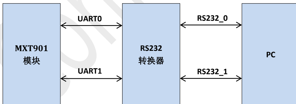
图 9-4 串口连接到 PC
