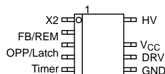
NCP1249C/D (Top View)
