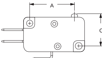
FIG. 2 Pin Roller
