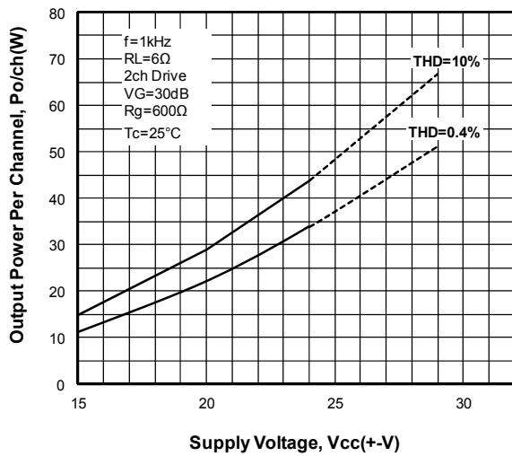
Po-Vcc
