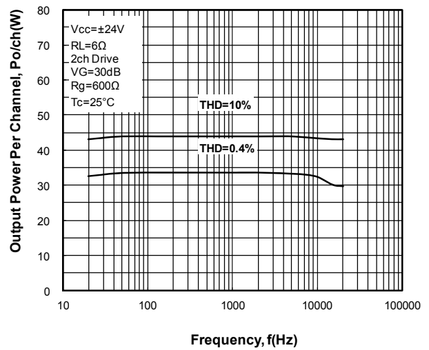
Po-f
