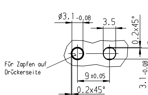
Empfohlenes Lochbild
