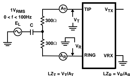
FIGURE 2. LONGITUDINAL IMPEDANCE
