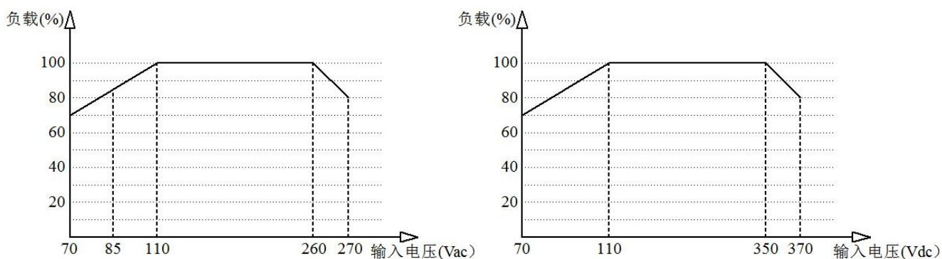
输入电压与负载特性曲线
