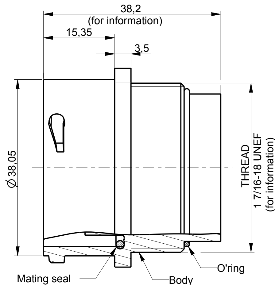
COUPE C-C
