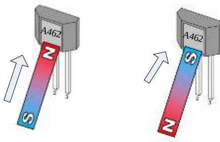
V_{OUT} =低电平
