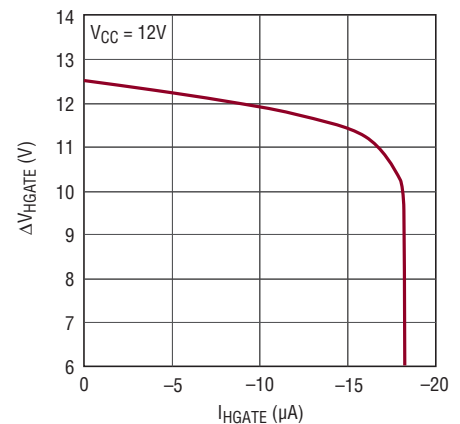
\Delta V_{\text{HGATE}} vs I_{\text{HGATE}}
