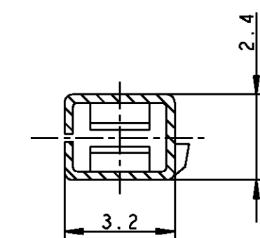
SEZ. (SECT.) B-B
