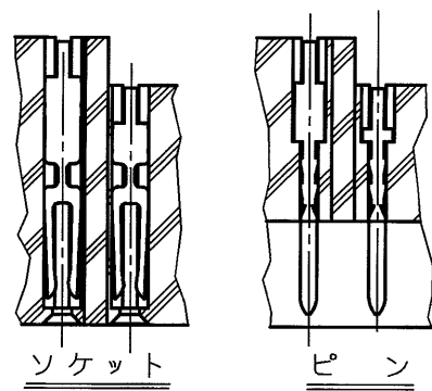
断面A-A (尺度 2:1)
