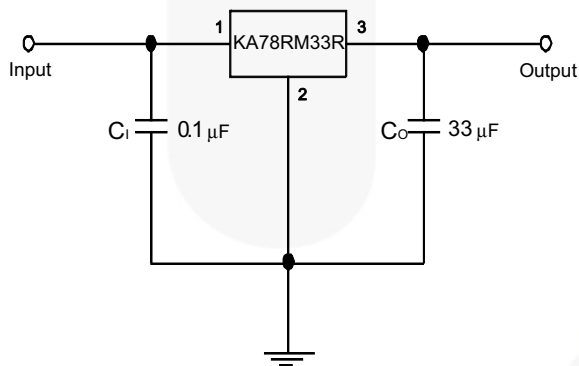
Figure 2. DC Parameters
