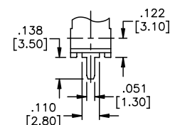
P.C. terminal
