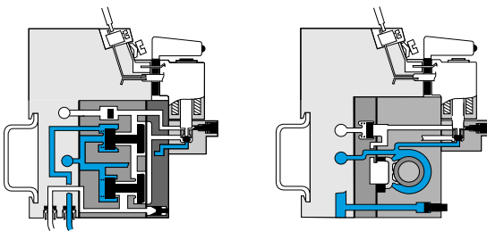
4/2 monostable module
