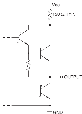
74OL6000/01 Output
