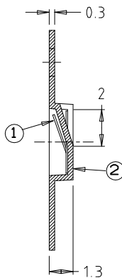
SECT.A-A
