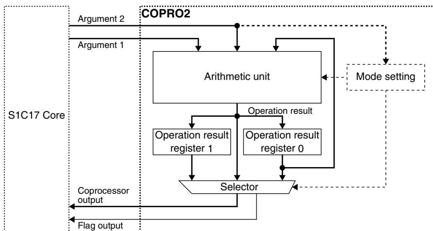
Figure 22.1.1 COPRO2 Configuration
