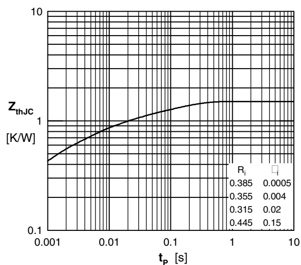
Fig. 6 Typ. transient thermal impedance
