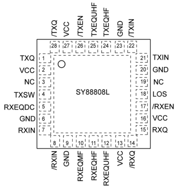
28-Pin QFN
