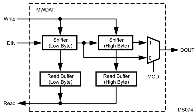
Figure 22-8. MWDAT Register
