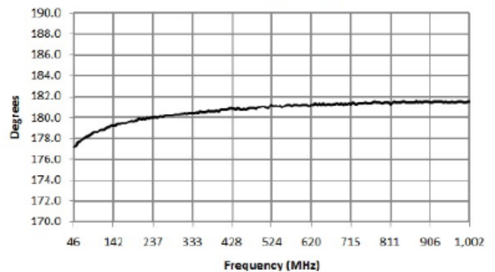
MABA-010245-CT1160 phase_balance
