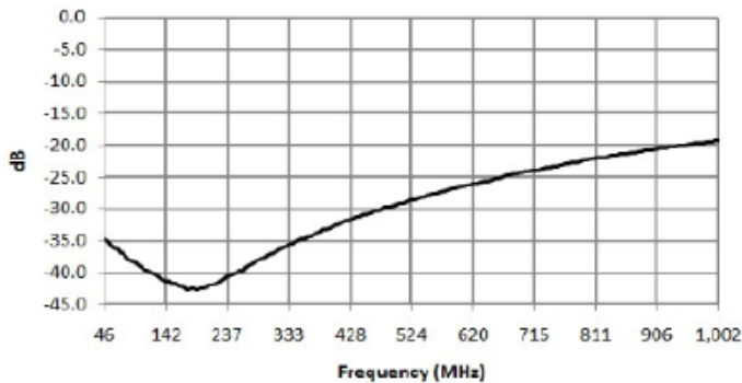
MABA-010245-CT1160 input_return_loss_pin_4
