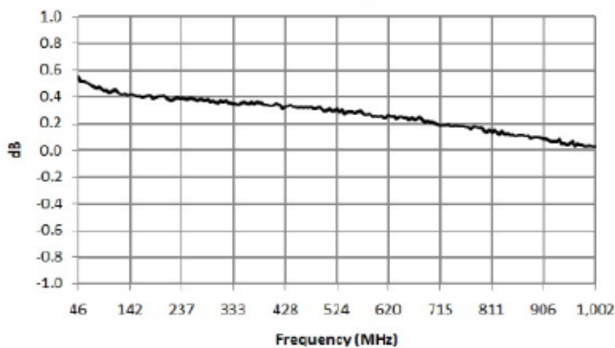
MABA-010245-CT1160 amplitude_balance
