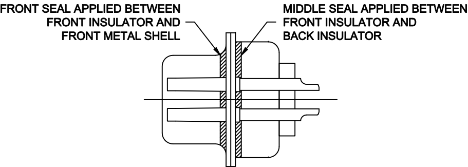
DETAIL A-A
