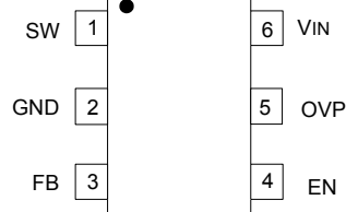
SOT26 / TSOT23-6
