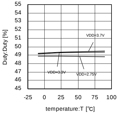
Fig.79 48MHz
