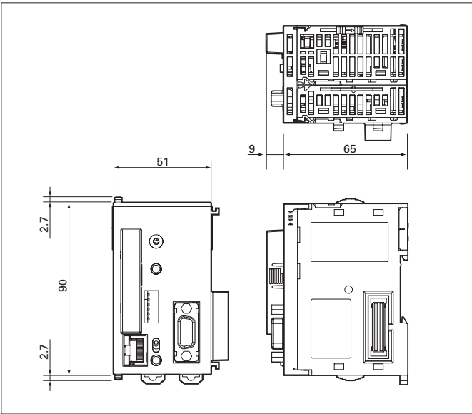
CJ1W-SPU01-V2
