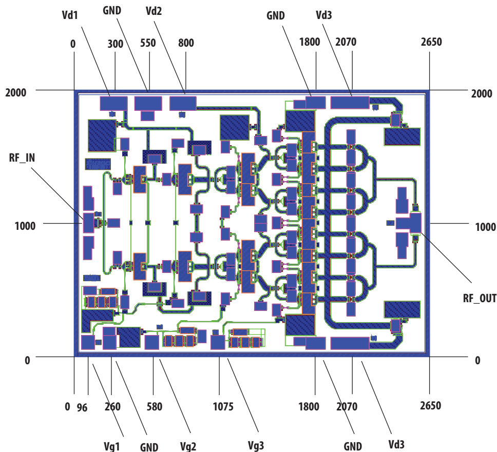
Figure 15. Die dimensions
