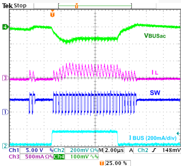
Figure 33. Load Transient, 5\text{-}155\text{-}5\text{ mA} , t_R=t_F=100\text{ ns}
