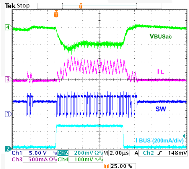
Figure 34. Load Transient, 5\text{-}255\text{-}5\text{ mA} , t_R=t_F=100\text{ ns}
