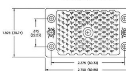
120 PIN RECEPTACLE
