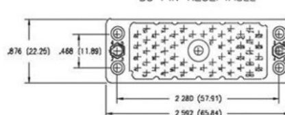
56 PIN RECEPTACLE
