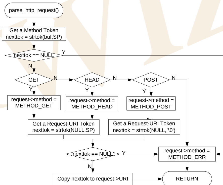
<Fig 3.20: parse_http_request() >
