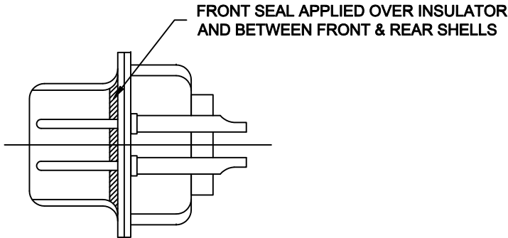
DETAIL A-A
