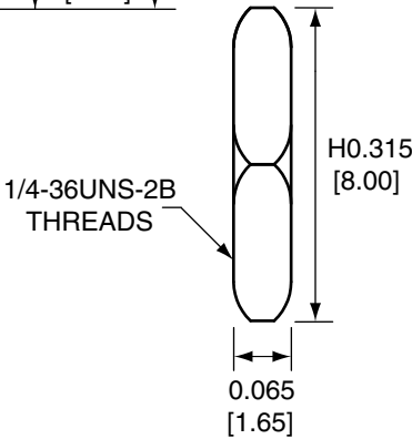
NUT
