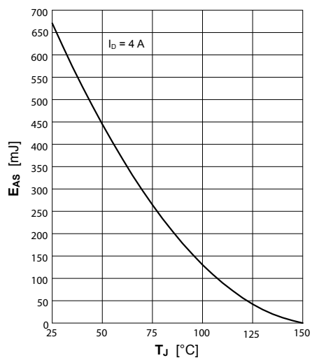
Fig. 10 Avalanche energy
