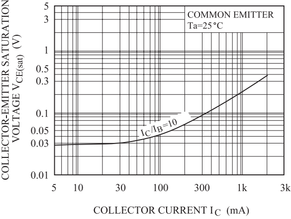
V_{CE(sat)} - I_C
