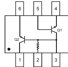
SOT26
