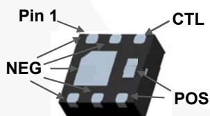
MicroFET2x2 mm
