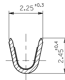
SECT.A-A
