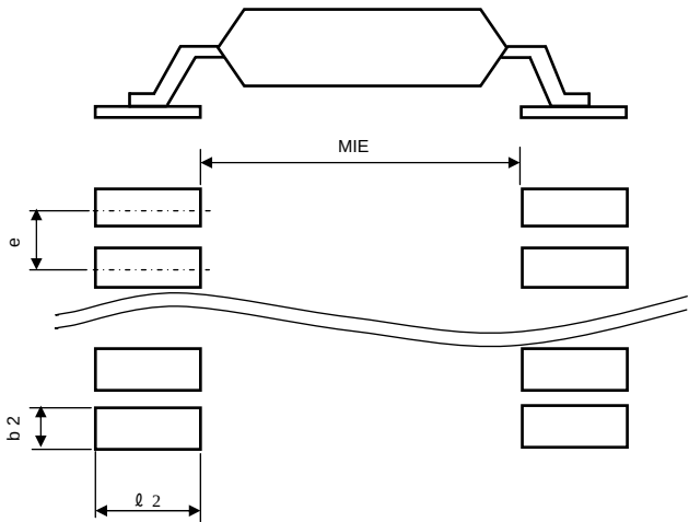
SOP8, SOP14, SSOP-B8 SSOP-B14, MSOP8
