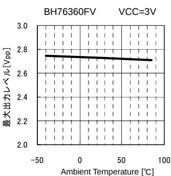
Fig.28 Vom vs. Ambient Temperature
