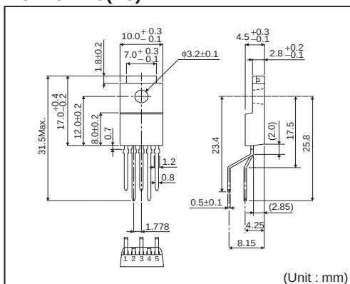
TO220FP-5(V5)
